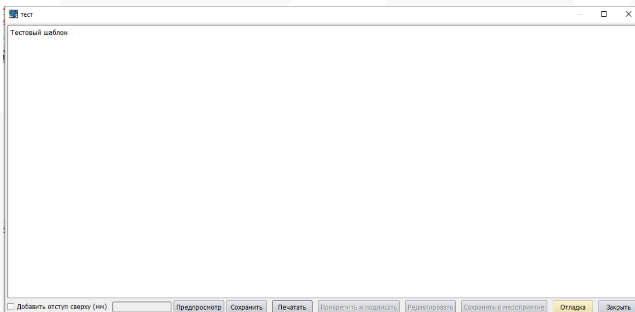
Рисунок 2 – Кнопка «Отладка»
