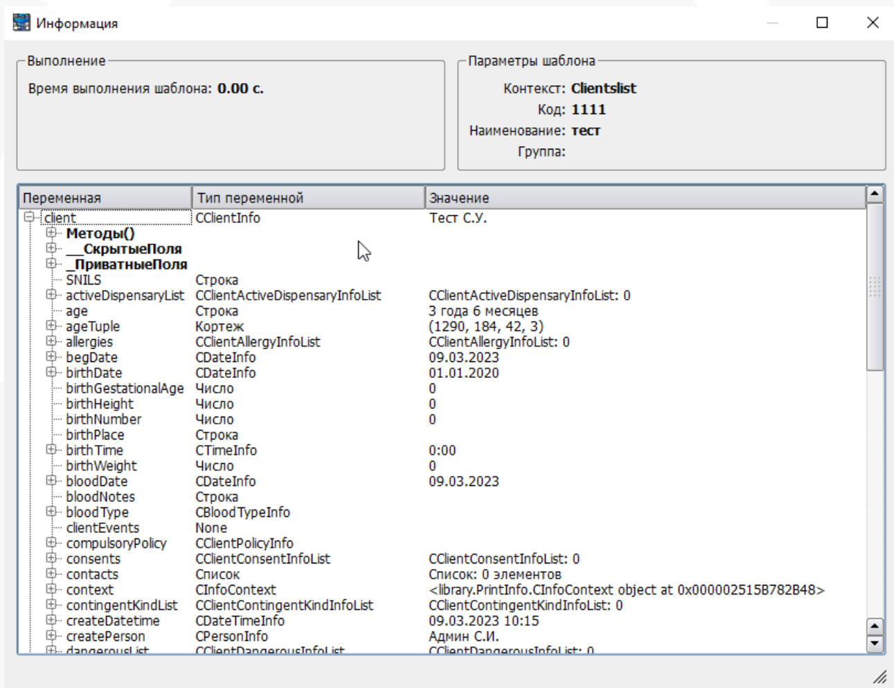
Рисунок 9 – Браузер атрибутов
